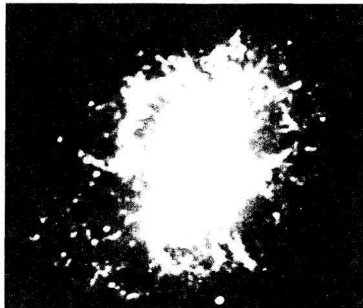
Крабовидная туманность, образовавшаяся после взрыва сверхновой звезды в 1054 году. В центре ее нейтронная звезда (пульсар) диаметром всего 25 км, хотя ее масса превышает массу нашего Солнца. Пульсар вращается со скоростью 30 оборотов в секунду и своей энергией питает туманность. «СЕРДЦЕ СПАСИТЕЛЯ» бьется уже 947 лет!
